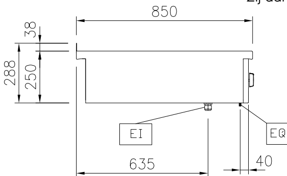
Zij aanzicht
