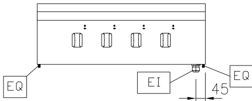
Front aanzicht
